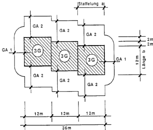
Abb. 2: lagemässig gestaffelte Baukörper
