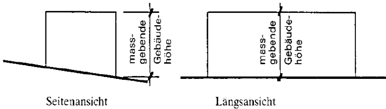
Abb. 6: Messen der Gebäudehöhe (§ 18 Abs. 2)
