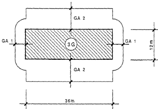
Abb. 1: einfache Baukörper
