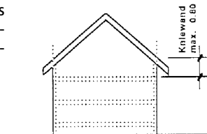
Abb. 3: Anrechenbarkeit des Dachgeschosses (§ 17 bis Abs. 1)
