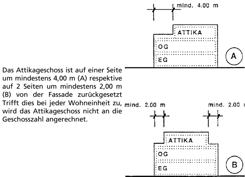
Abb. 4: Anrechenbarkeit des Attikageschosses (§ 17 bis Abs. 3)
